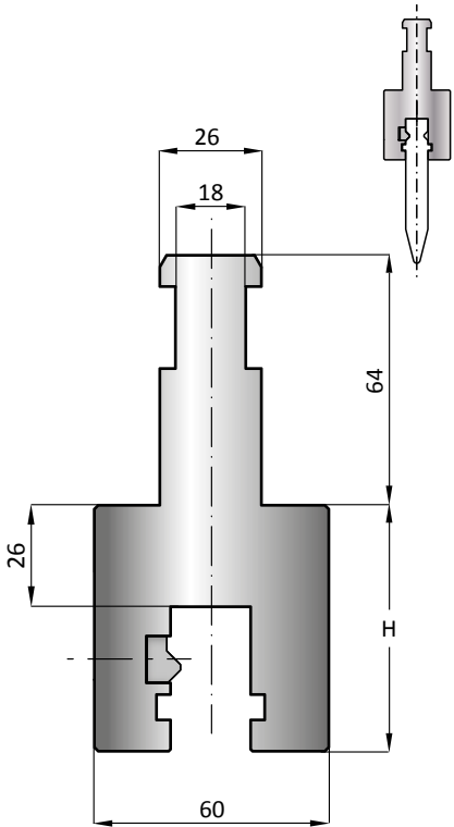
ADATTATORE- ADAPTER - ADAPTADORE ADAPTADORE - ADAPTATEUR - ADAPTER EHT / WILA - TRUMPF
